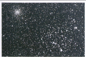
Рассеянное скопление M35 в созвездии Близнецов. Содержит несколько тысяч звезд. Видимая яркость 5.3 звездной величины.
