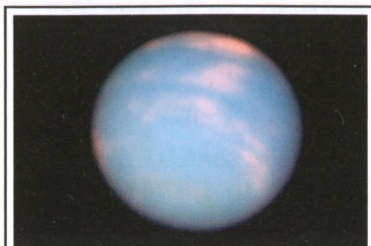
12 июля 2011 г. телескоп Хаббл отметил этим снимком Нептуна первый его оборот вокруг Солнца с момента открытия планеты 165 лет назад.
