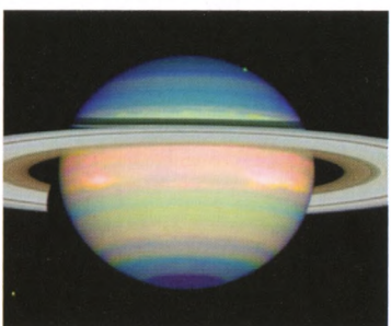
Сатурн в ложных ярких цветах. Снимок сделан инфракрасной камерой (NICMOS) космического телескопа Хаббл 4 января 1998 г. и показывает отраженный планетой инфракрасный свет. Это позволяет получить подробную информацию об облачности Сатурна.
