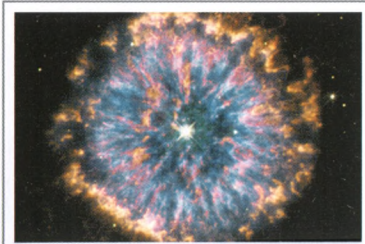
Планетарная туманность NGC 6751 в созвездии Орла напоминает зрачок глаза. Снимок получен с помощью телескопа Хаббл.
