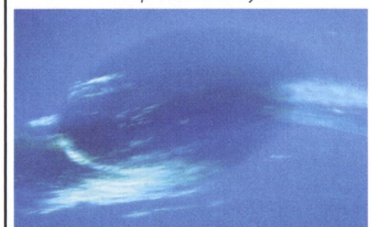
Снимок Большого Темного Пятна Нептуна, сделанный КА Вояджер с расстояния 2,8 миллиона километров 30 августа 1999 г. На снимке можно различить объекты минимальной протяженностью до 50 км.
